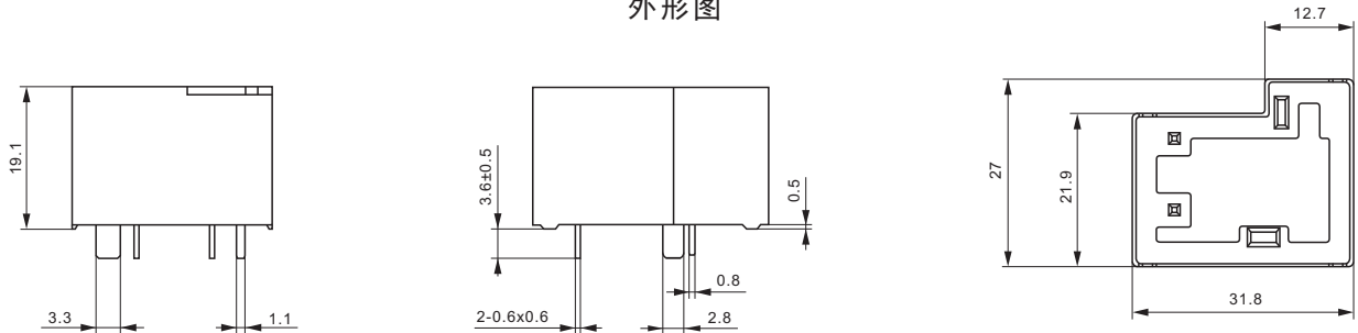
外形图
